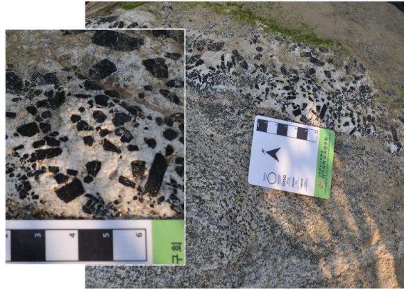
탐구지점3-B1 : 수로 주변 암석
